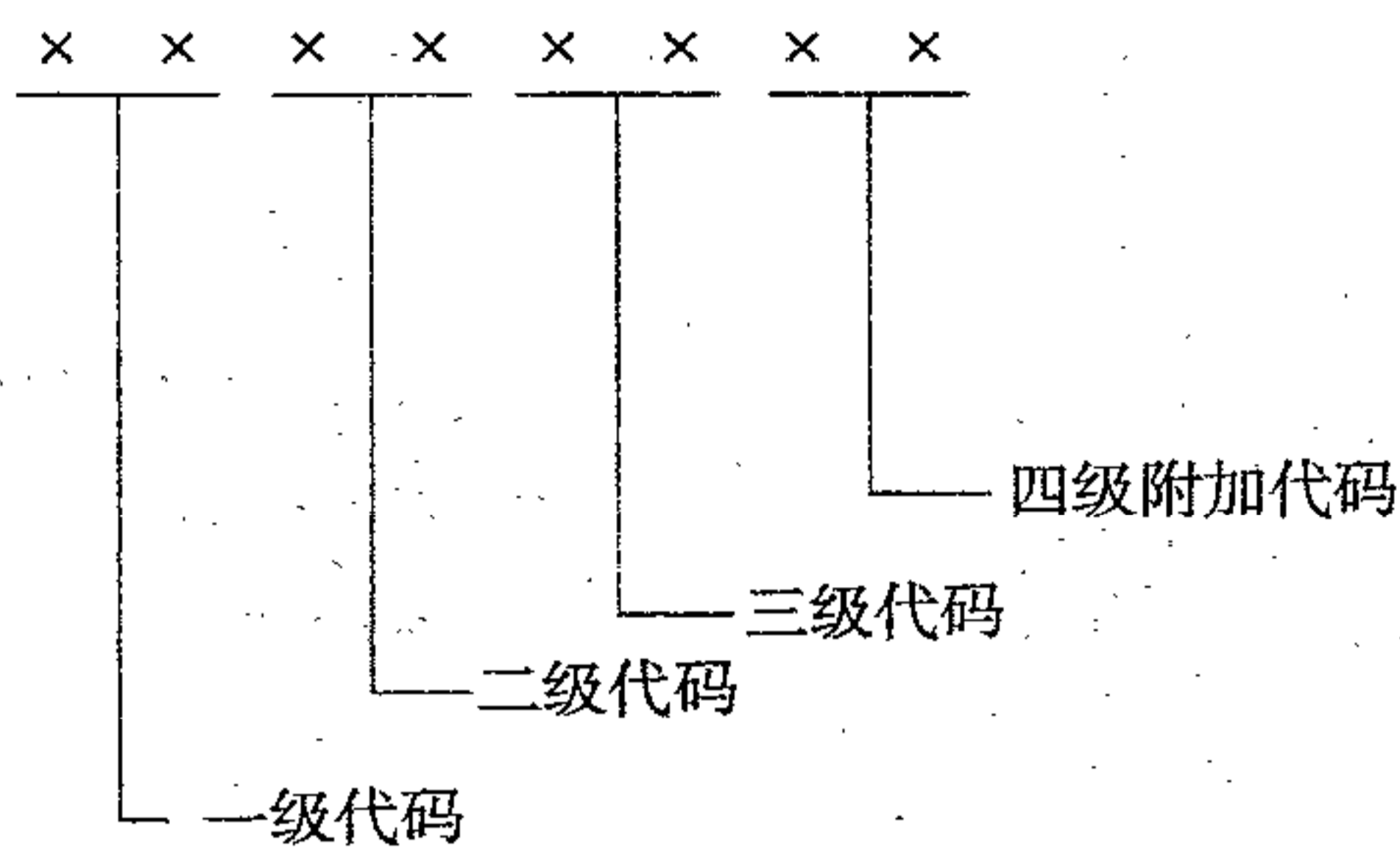
图 1 代码结构
